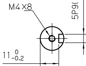
軸端部詳細
