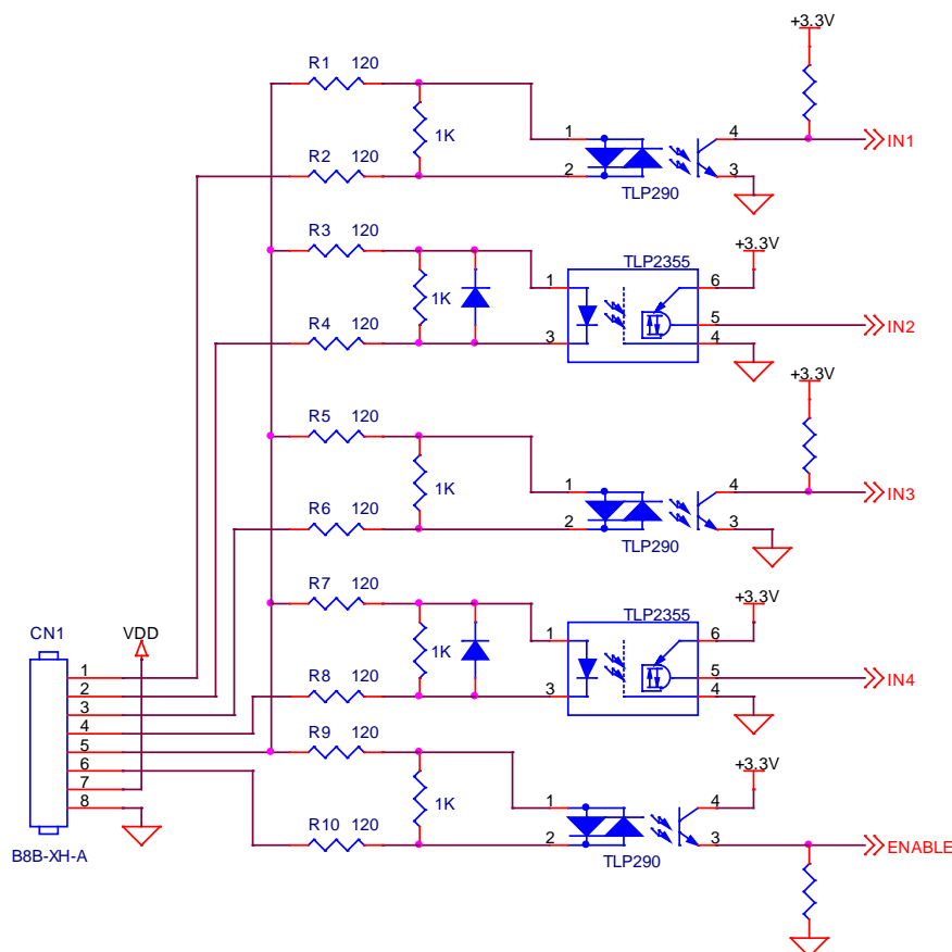
図 4.2 信号受信回路
