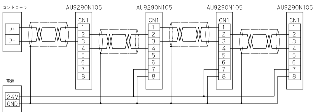
図 4.3 RS485 シリアルバスの接続例
