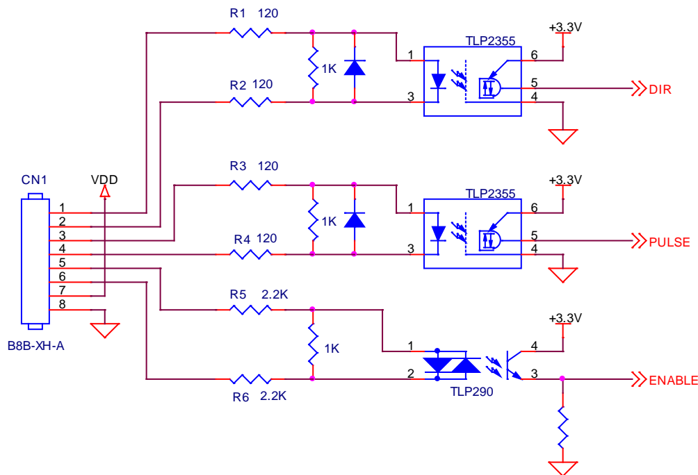
図 4.1 信号受信回路
