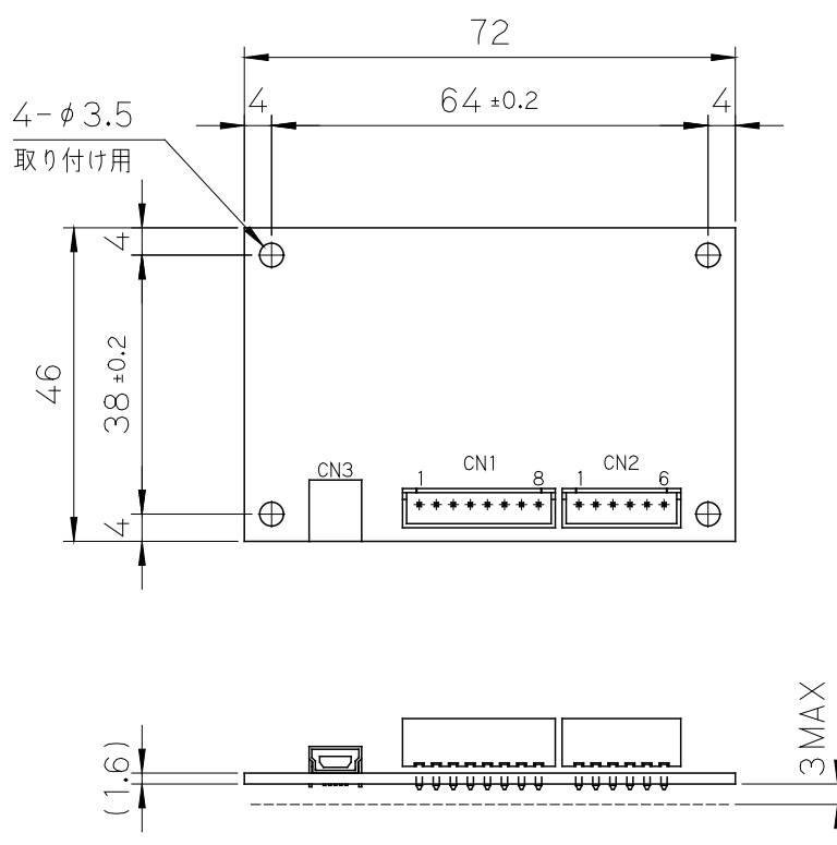
図 14.1 AU9290N10x 外形図
