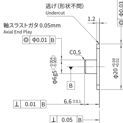
モータ取付推奨寸法 Recommended Dimension of the Motor Shaft
