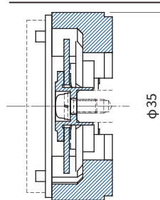
断面 D-O-D Sectional Plan DOD
