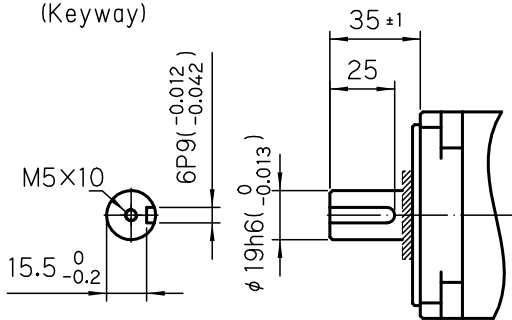
軸端部詳細
