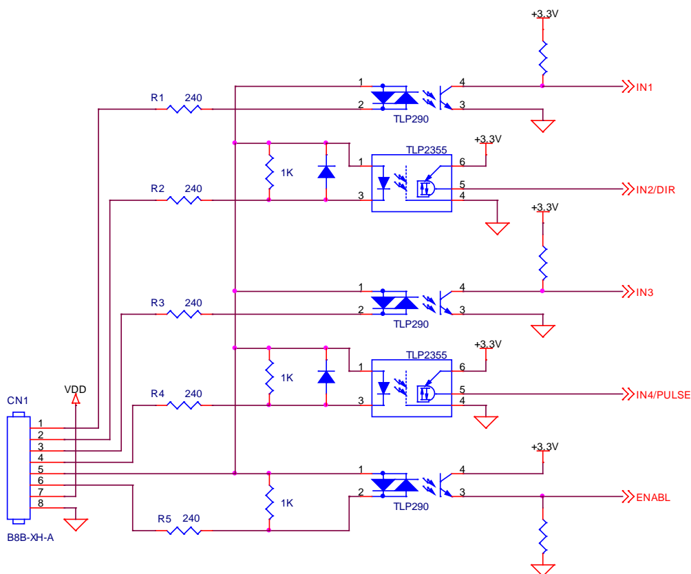
図 4.1-2 受信回路 (AU9290N103 と AU9290N104 の場合)
