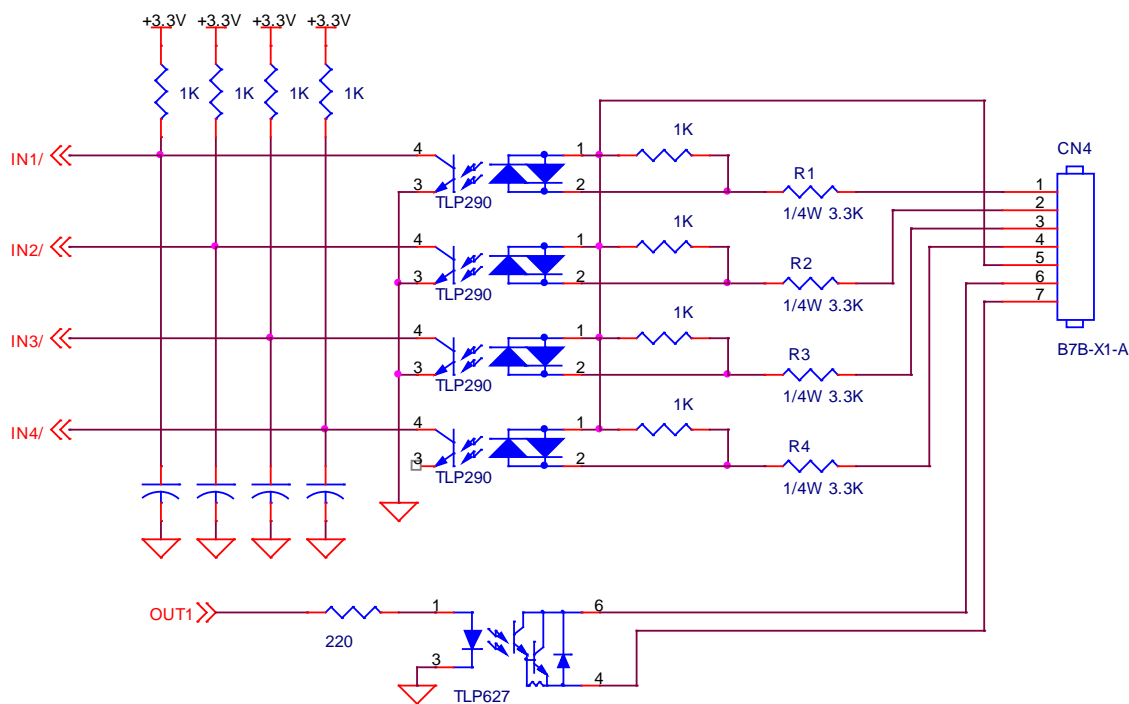
図 4.2 平行 I/O 信号の入出力回路
