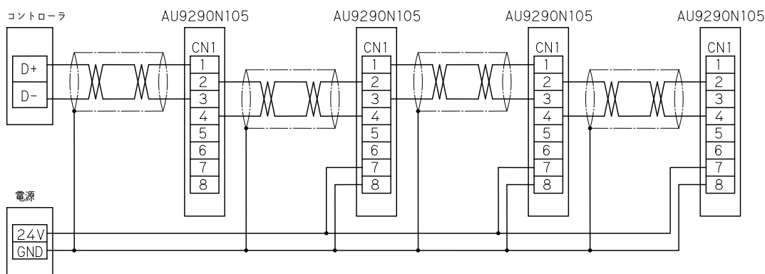
図 4.1-3 RS485 シリアルバスの接続例
