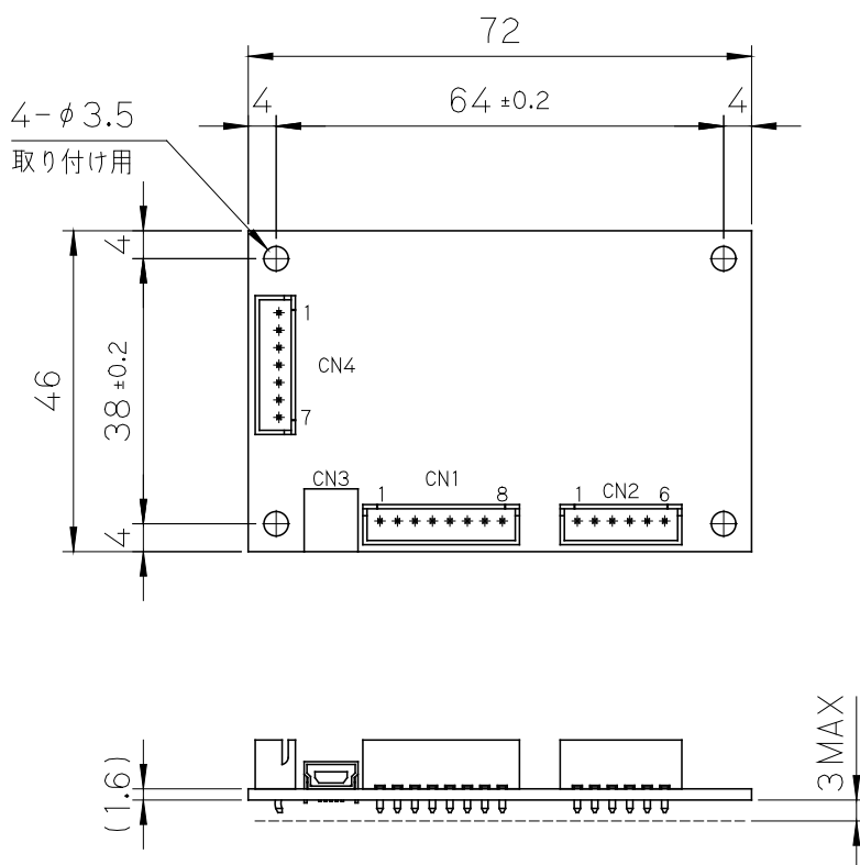
図 14.1 AU9290 外形図
